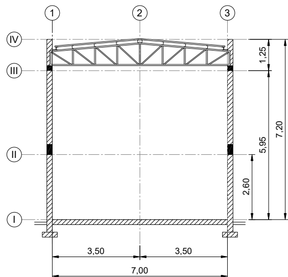
Sección
